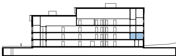
Řez
